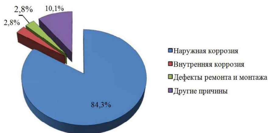
Рис. 1. Статистические данные о причинах аварийных ситуаций на тепловых сетях
