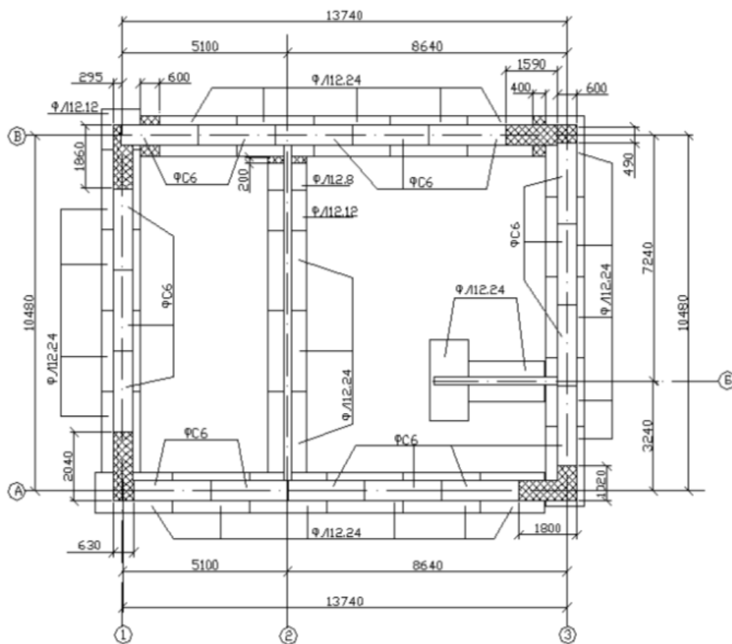
План фундамента
