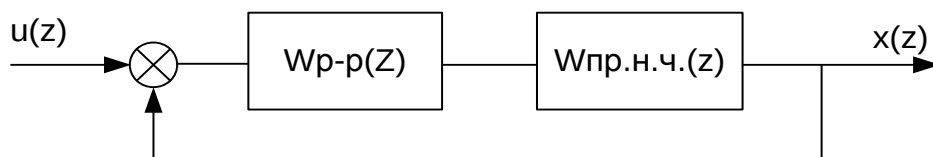
Рисунок 3.5 – Эквивалентная дискретная система
