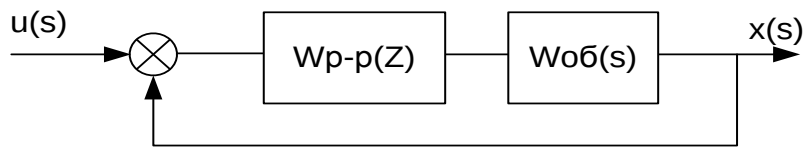
Рисунок 3.3 - Дискретно-непрерывная одноконтурная система
