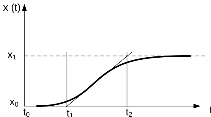
Рисунок 3.2 – Расчет параметров объекта по кривой отклика
