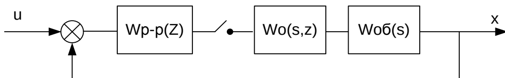
Рисунок 3.4 – Структурная схема, иллюстрирующая преобразование непрерывного сигнала
