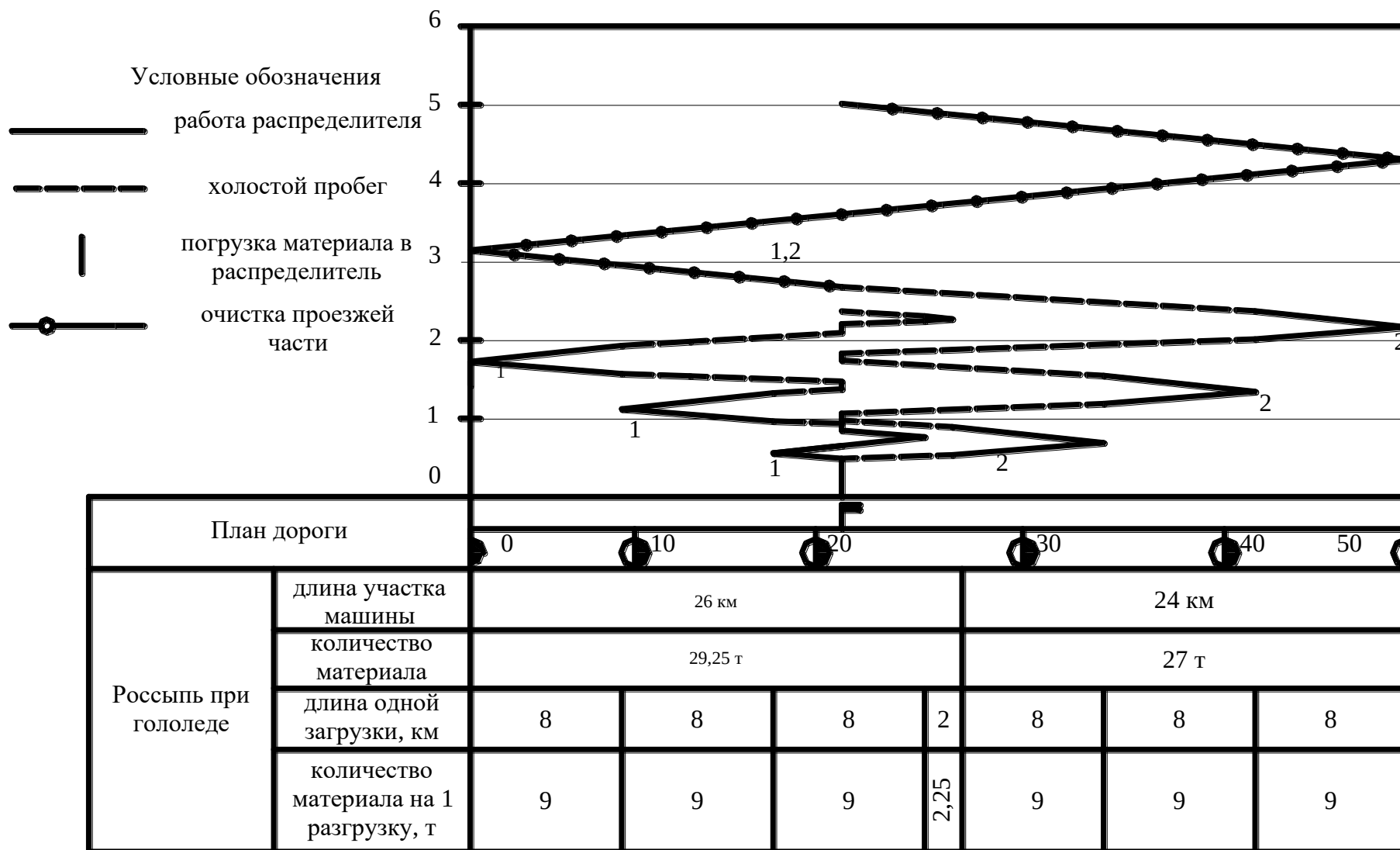
Рисунок 6 – График работы распределителей противогололедных материалов (пример)
