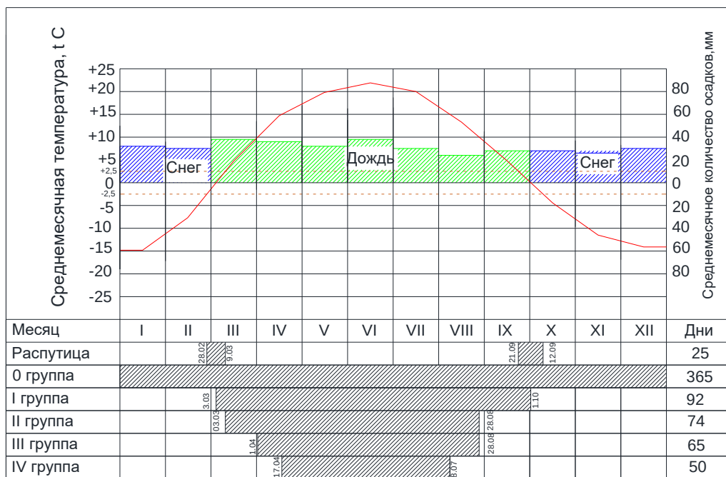
Рисунок 1 – Дорожно-климатический график
