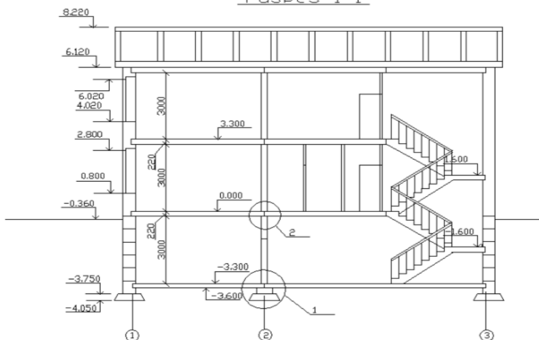
Разрез 1-1
