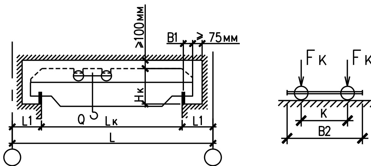
Рис. 2 – Габариты крана
