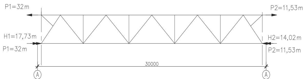
Рис. 20 – Схема приложения распоров и сосредоточенных сил
