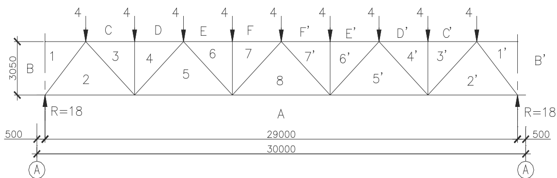
Рис. 22 – Схема приложения вертикальной снеговой нагрузки
