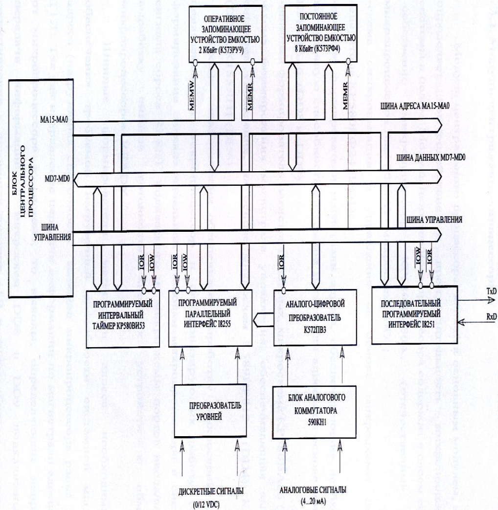
Рис. 2.1. Структурная схема микропроцессорной системы контроля
