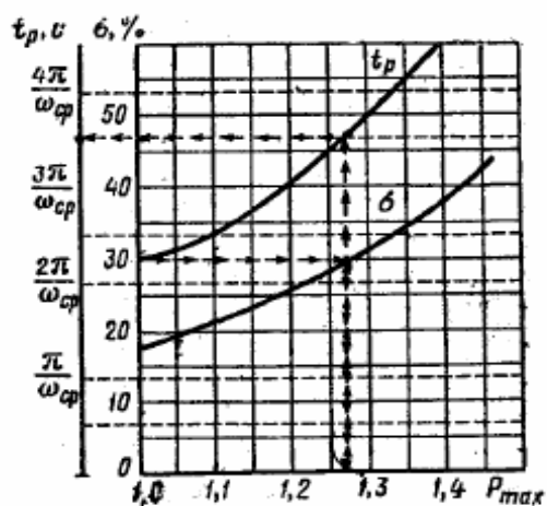
Рисунок Г.1- График для определения P_{max} и частоты среза по заданному перегуливанию \sigma
