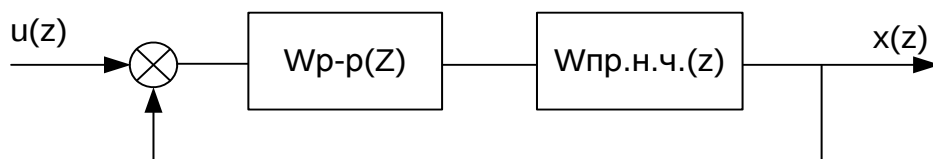
Рисунок 3.5 – Эквивалентная дискретная система
