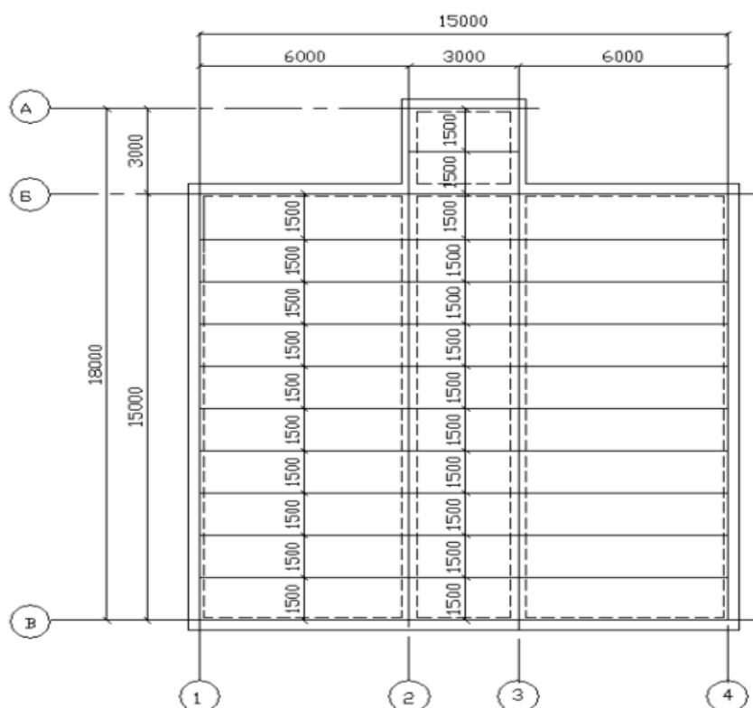
План перекрытия
