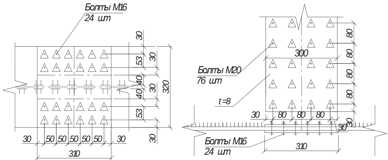
Рис. 2.12 – Расстановка болтов
