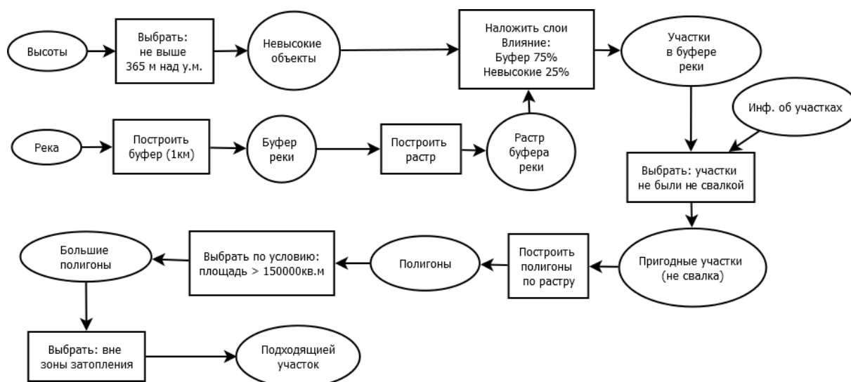
Рисунок П6.1. Алгоритм ГИС анализа для определения оптимального местоположения новой водоочистной станции
