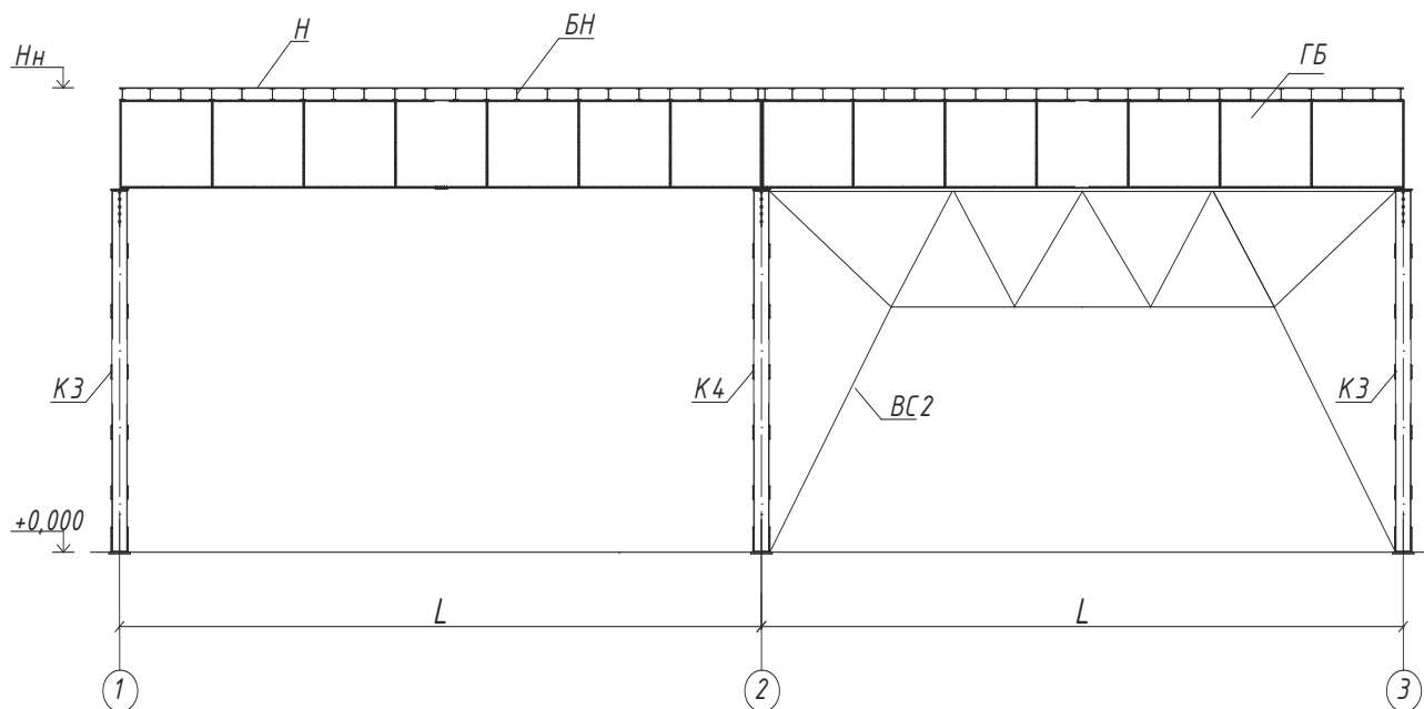
Разрез 1-1
